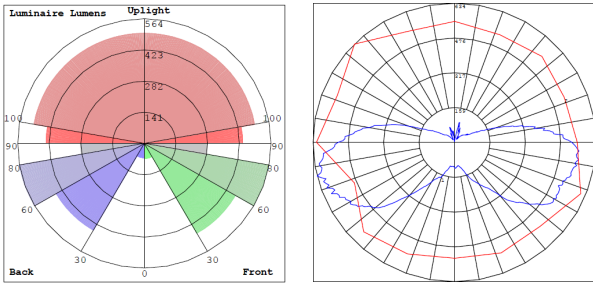
BUG Rating: B2-U3-G3
